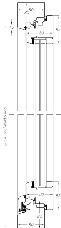
Sezione A-A'
